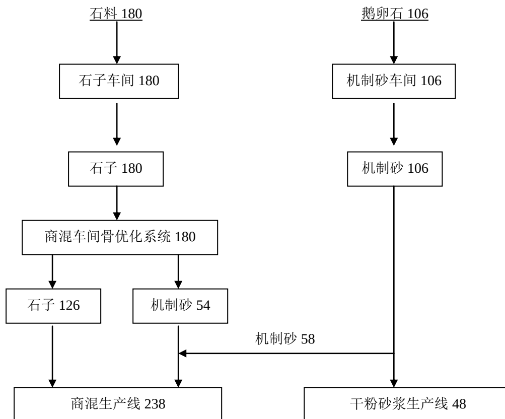
附图一 全场物料流动示意图（万 t）
