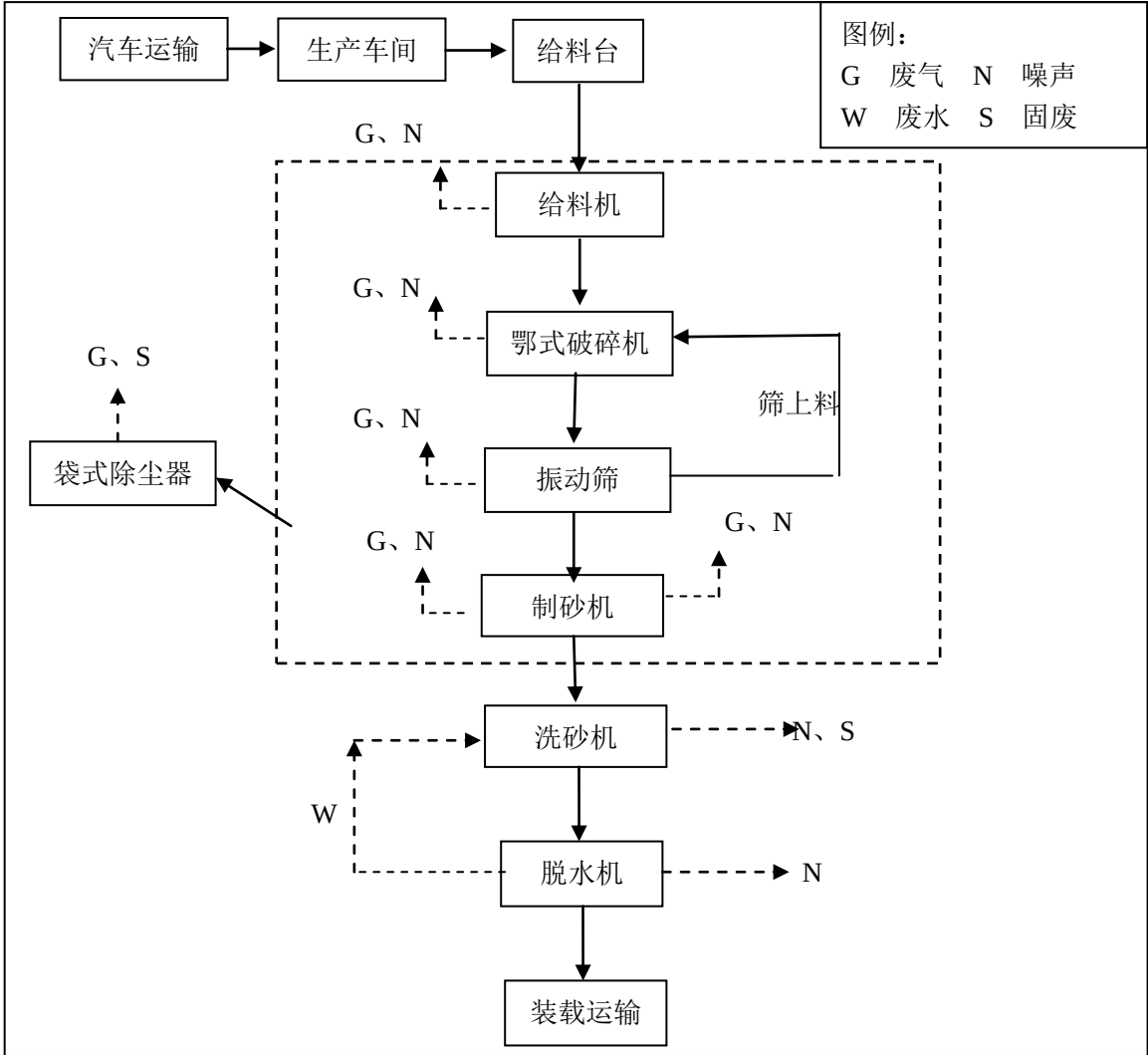
图五 机制砂生产工艺流程及产污环节示意图
