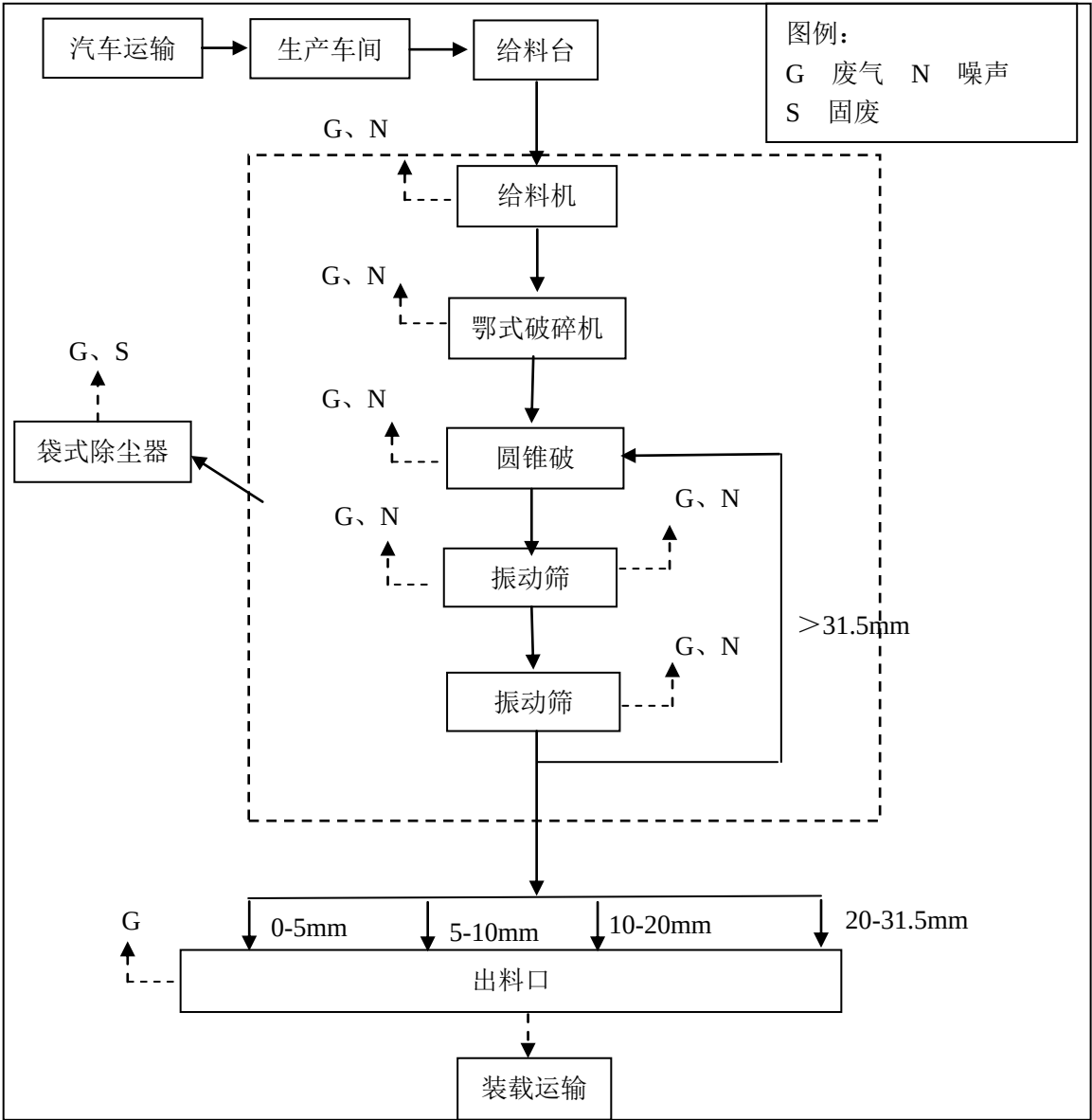
图四 石子生产工艺流程及产污环节示意图
