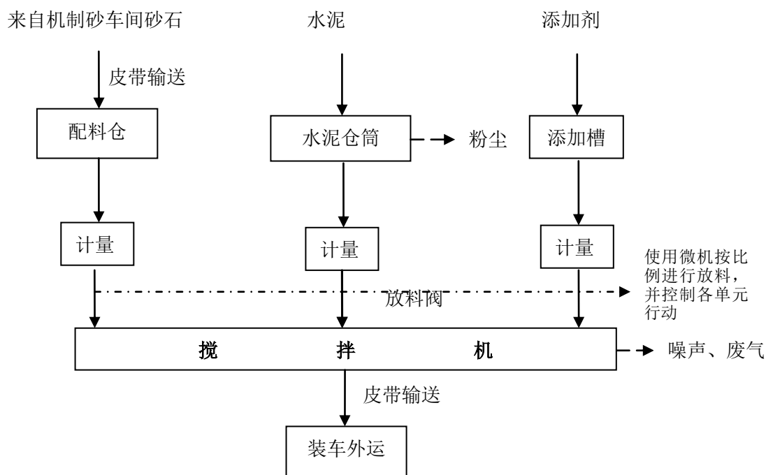
图三 干粉砂浆生产工艺流程图
