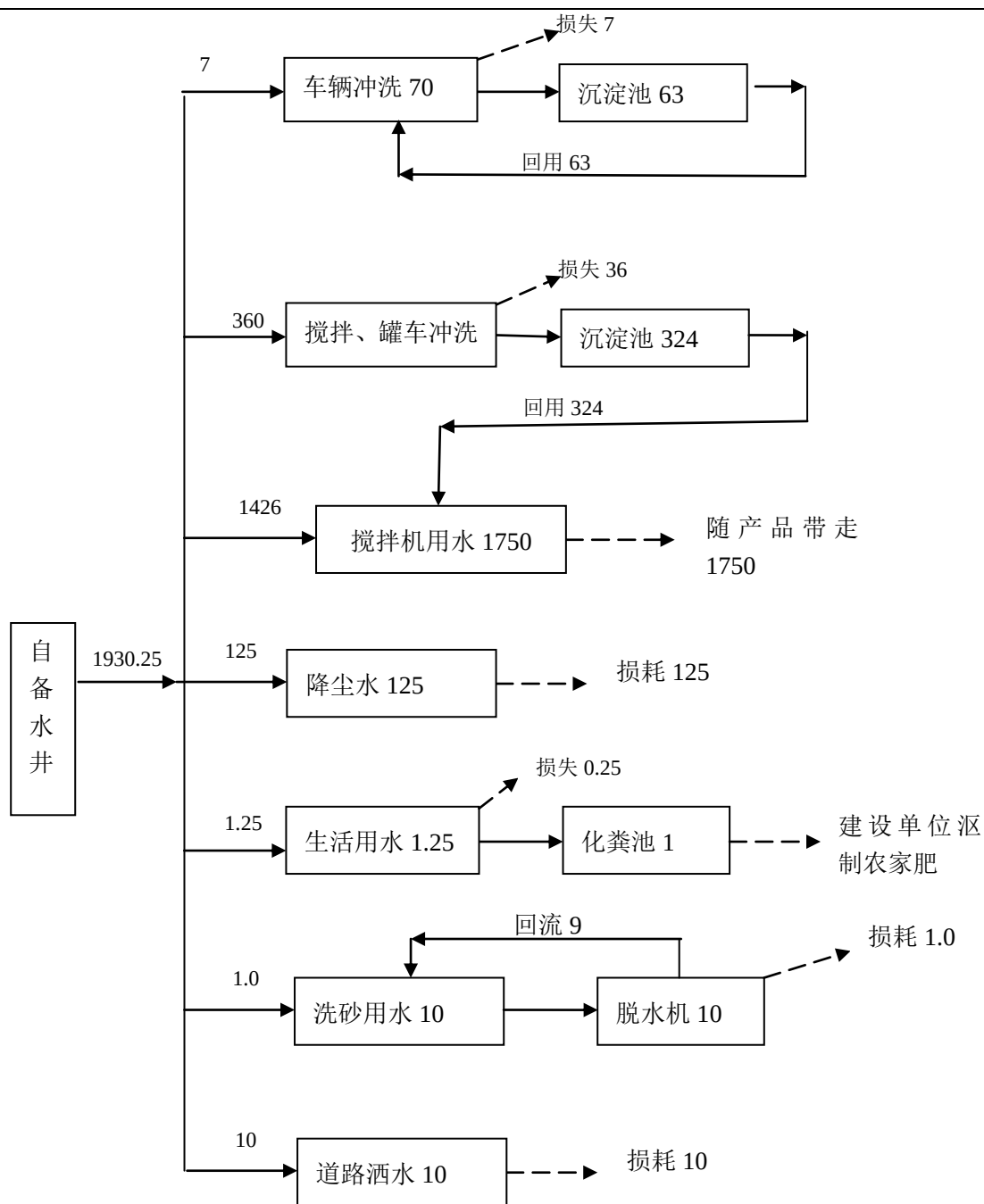
图六 本项目水量平衡图 (m³/d)
