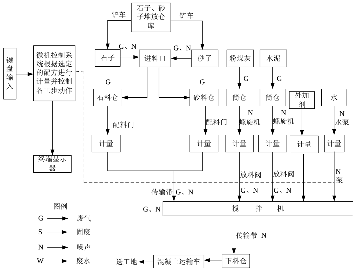
图二 商混生产工艺流程图
