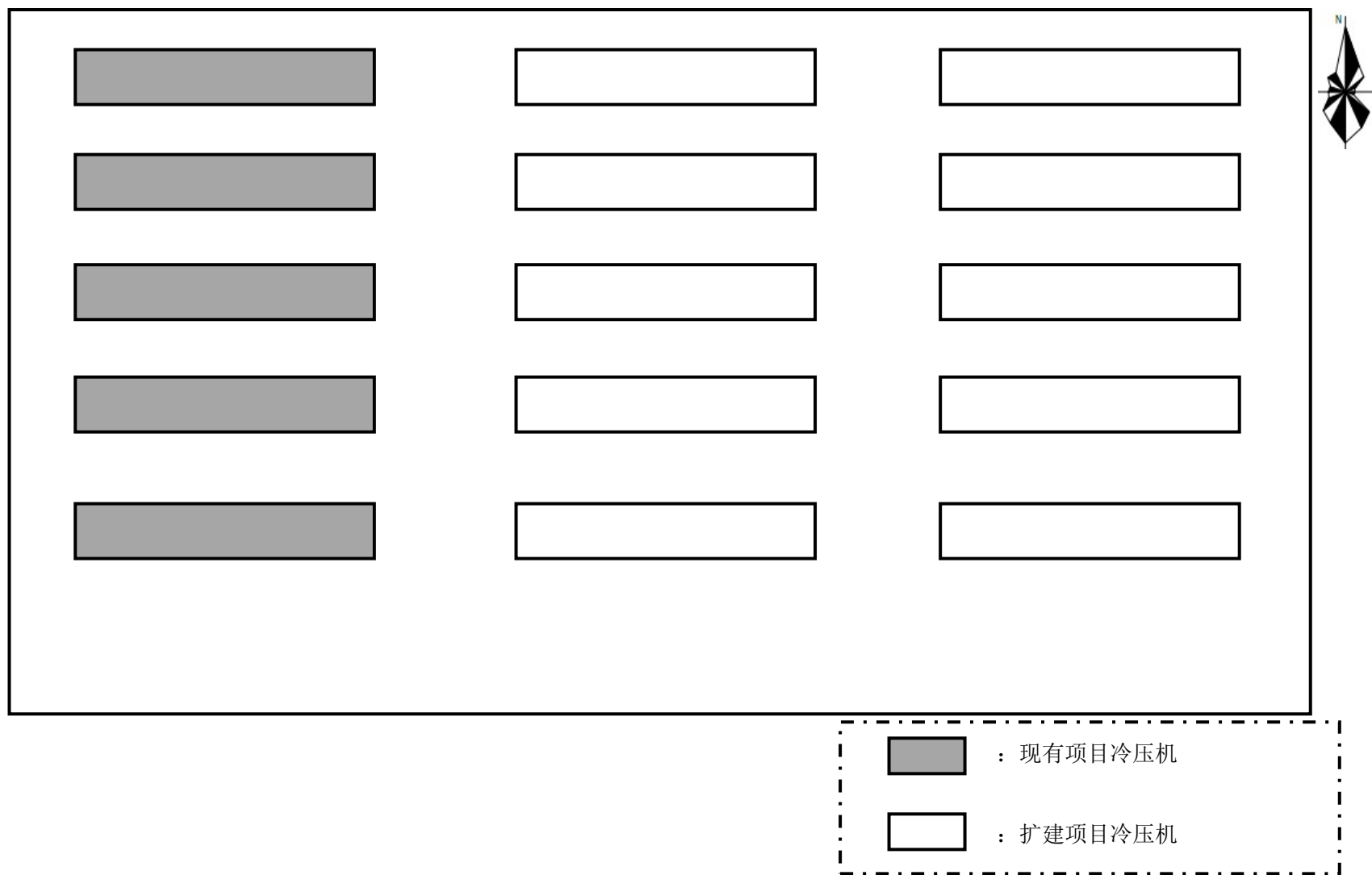
附图 3-2 项目生产车间平面布置图
