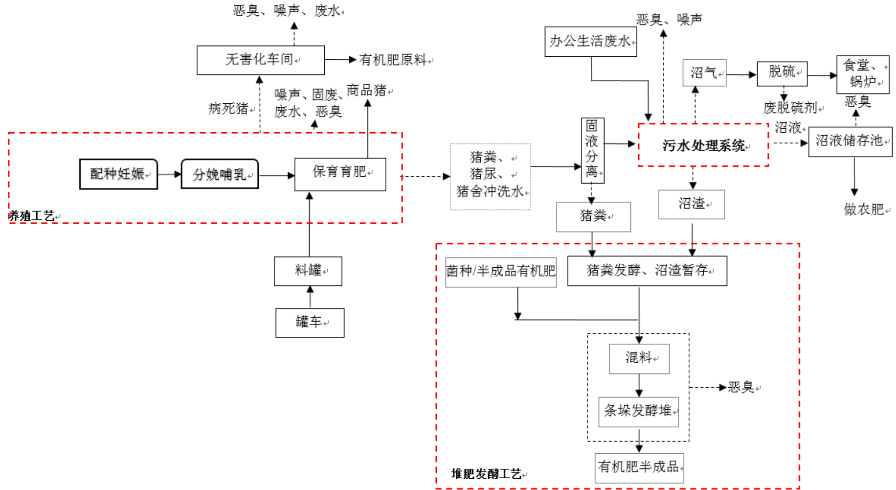
图 2-11 本项目运营期整体工艺及产排污环节图
