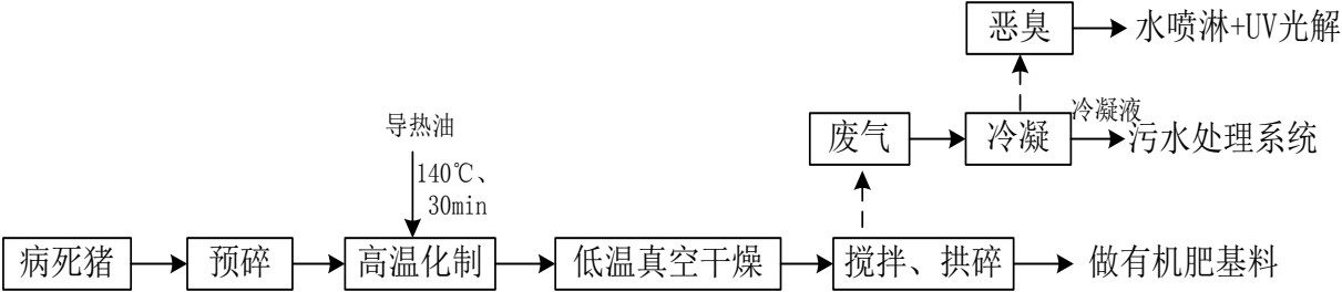
图 5-8 本项目病死猪无害化处理工艺流程图
