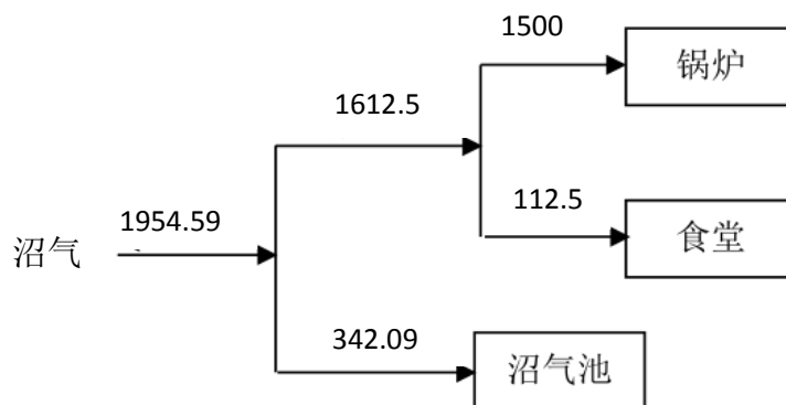
图 2-7 夏季沼气利用平衡图 (单位: \text{m}^3/\text{d} ) 122 天
