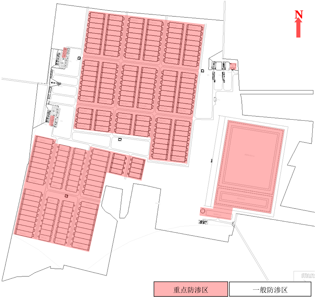
图 5-10 场区分区防渗示意图
