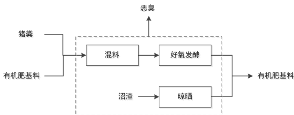
图 2-10 粪污发酵堆肥工艺流程及产污环节图
