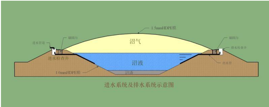
图 5-6 沼气工程进水系统及排水系统示意图
