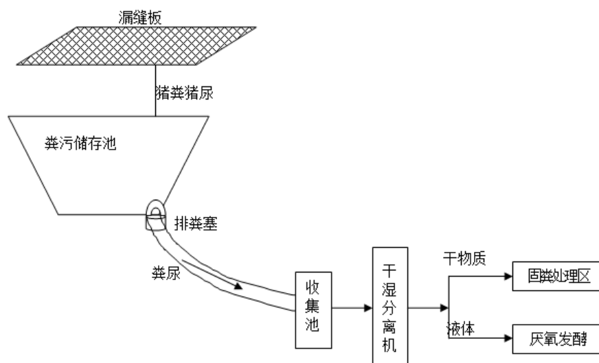
图 5-1 本项目清粪工艺示意图
