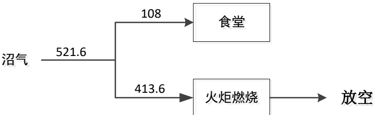
图 2-8 其他季节沼气利用平衡图单位：m 3 /d，243 天
