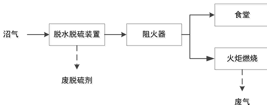
图 2-6 沼气利用流程及产污环节图
