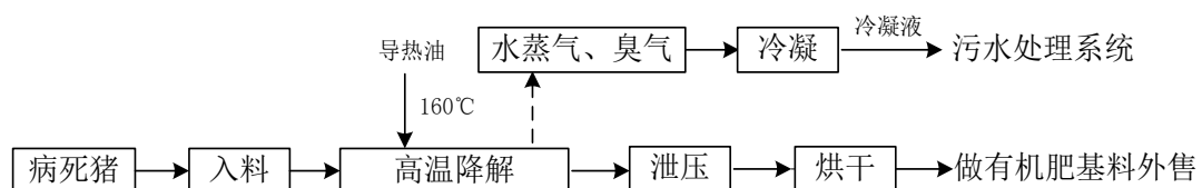
图 5-9 本项目病死猪无害化处理工艺流程图
