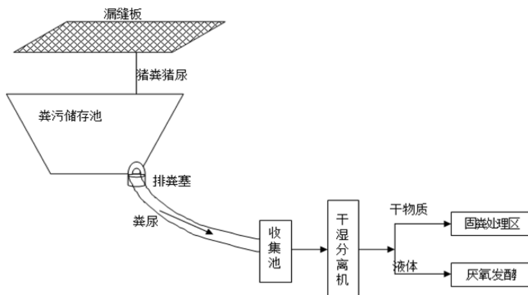
图 2-4 本项目清粪工艺示意图
