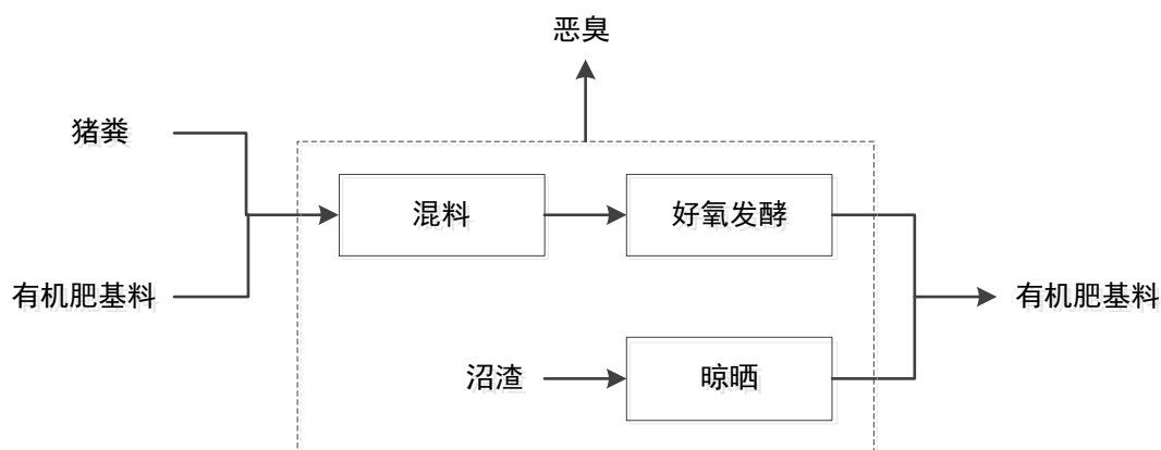
图 2-9 固粪处理区工艺流程及产污环节图
