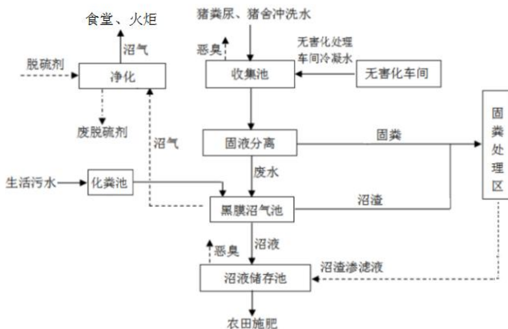
图 5-3 项目污水处理工艺流程图
