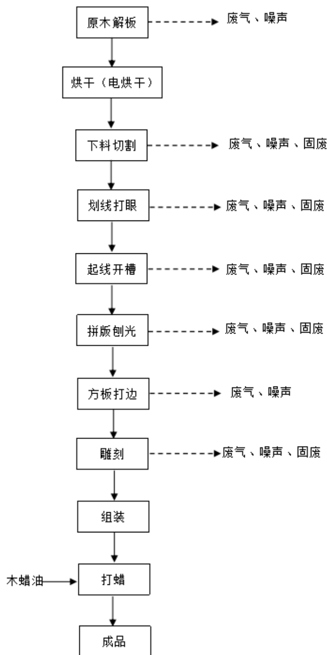
图 4 营运期生产工艺流程图
