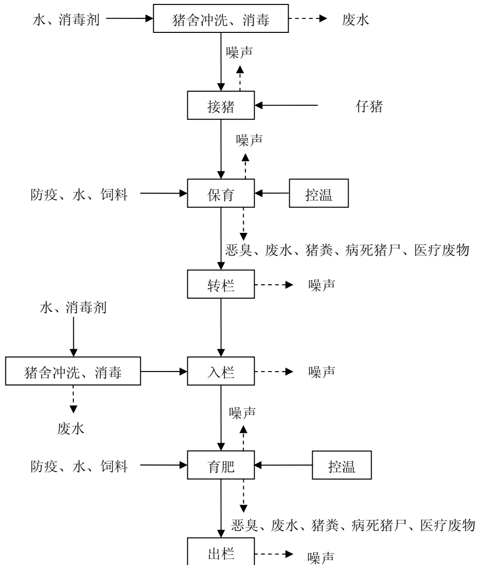
图 2-4 保育、育肥养殖过程工艺流程及产污环节图
