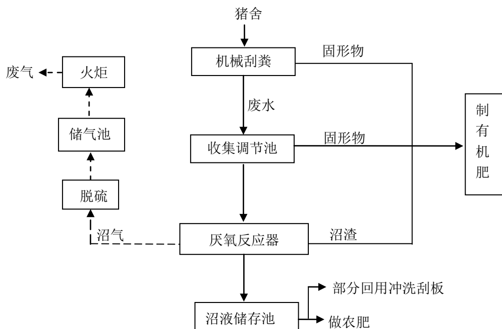
图3 现有工程污水处理工艺流程及产污环节图
