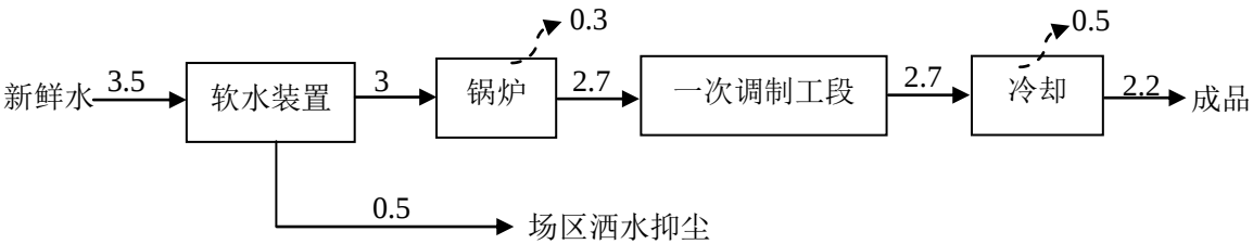
图 1 本项目水平衡图 散发量 单位：m³/d
