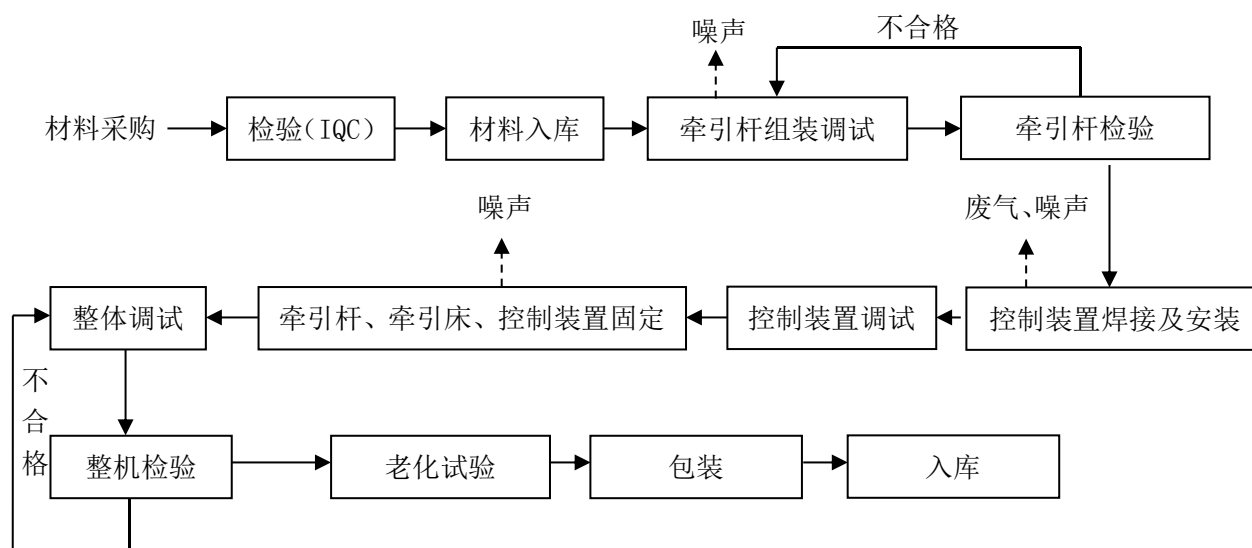
图 1 牵引床生产工艺流程图
