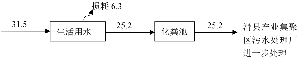
图 2 水平衡图 单位 m 3 /a
