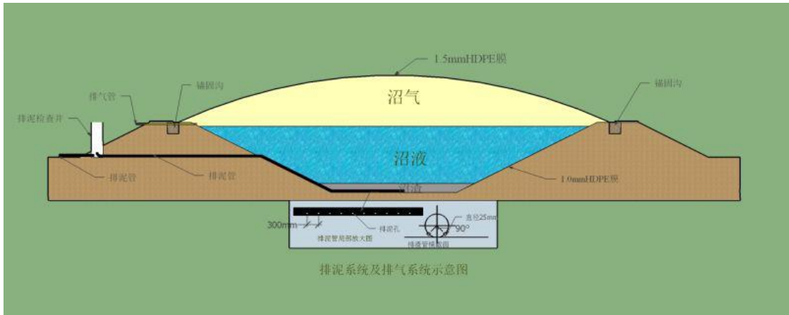
图 5-7 沼气工程排泥系统及排气系统示意图
