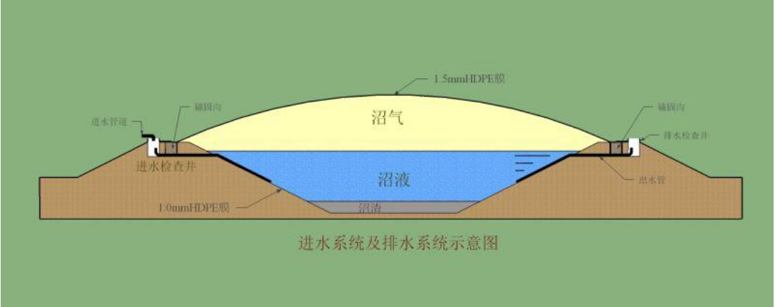
图 5-6 沼气工程进水系统及排水系统示意图
