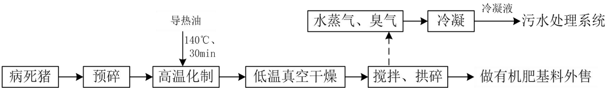
图 5-8 本项目病死猪无害化处理工艺流程图
