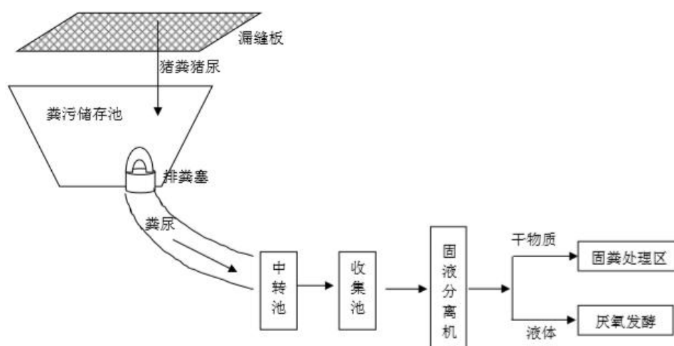
图 2-4 本项目清粪工艺示意图
