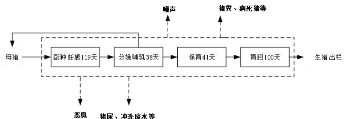
图 2-3 养殖过程工艺流程及产污环节示意图
