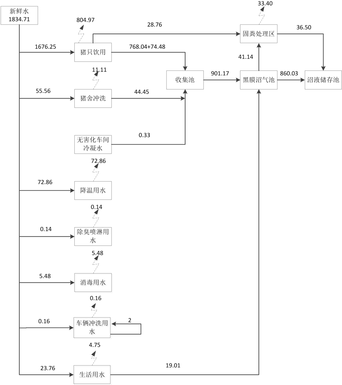
图 2-1 夏季水平衡图 单位 t/d
