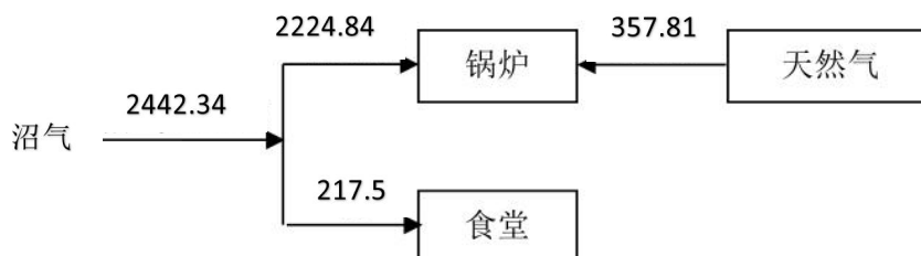
图 2-8 其他季节沼气利用平衡图 (单位: \text{m}^3/\text{d} ) 243 天
