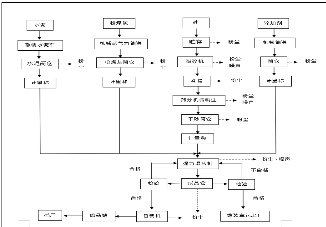
图二 生产工艺流程图
