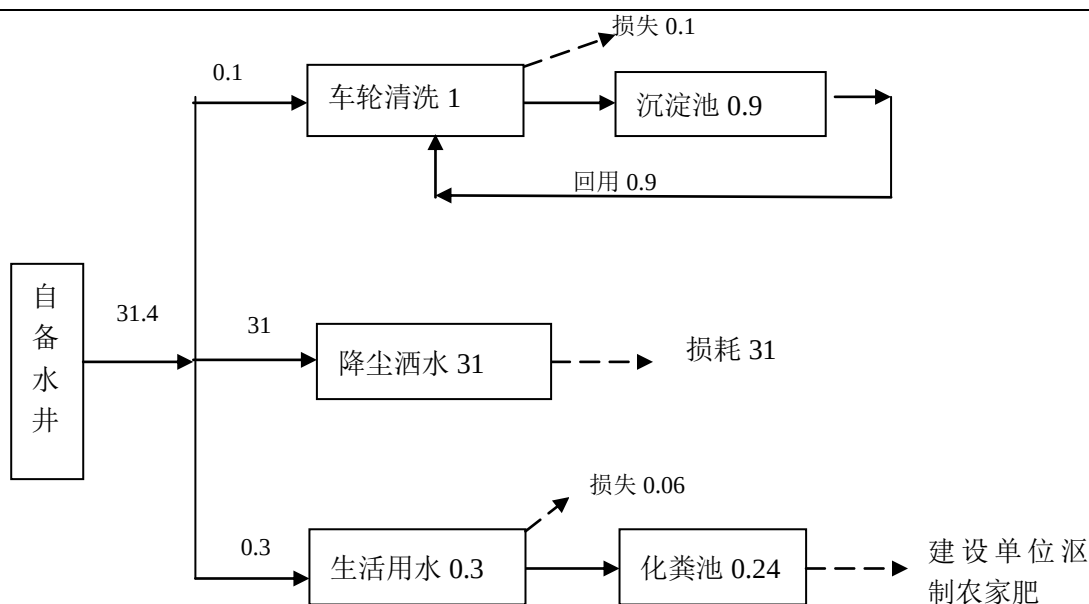
图三 本项目水量平衡图 (m 3 /d)
