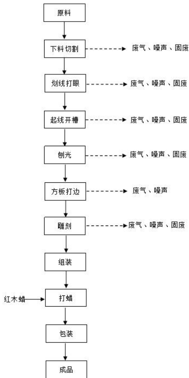
图 3：工艺流程图
