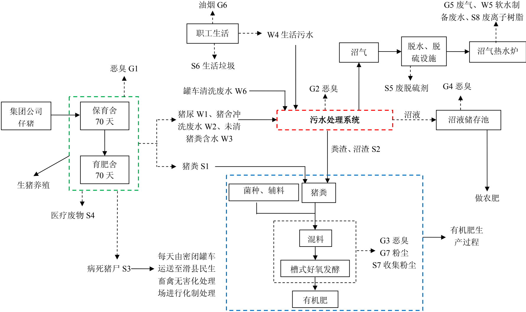
图 2-7 产污环节图
