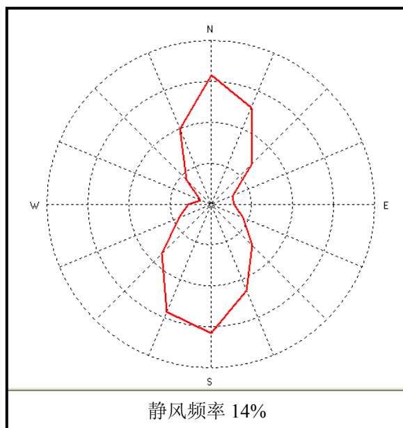
图 4-1 多年风向玫瑰图
