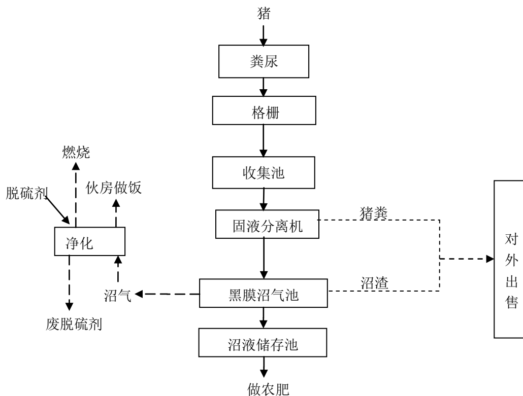
图 3 现有工程污水处理工艺流程及产污环节图
