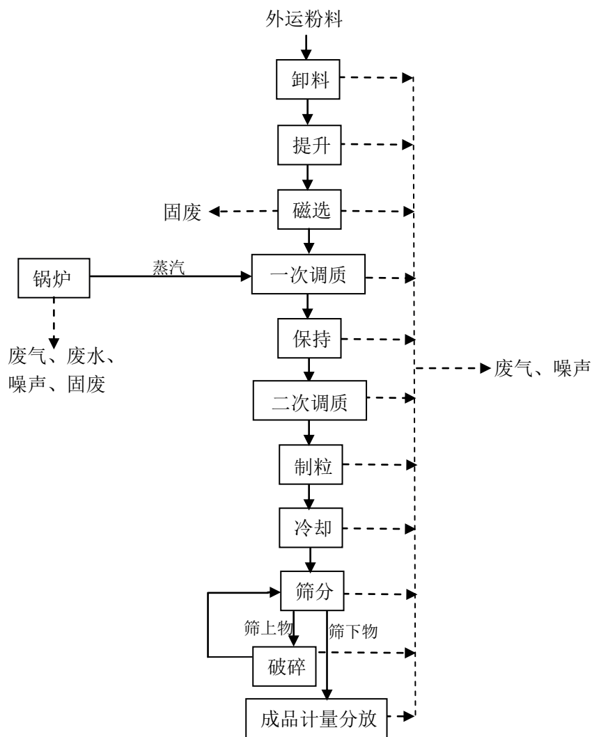
图 5 营运期工艺流程及产污环节图
