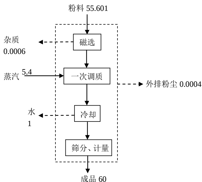
图 6 本项目物料平衡图 单位：t/d
