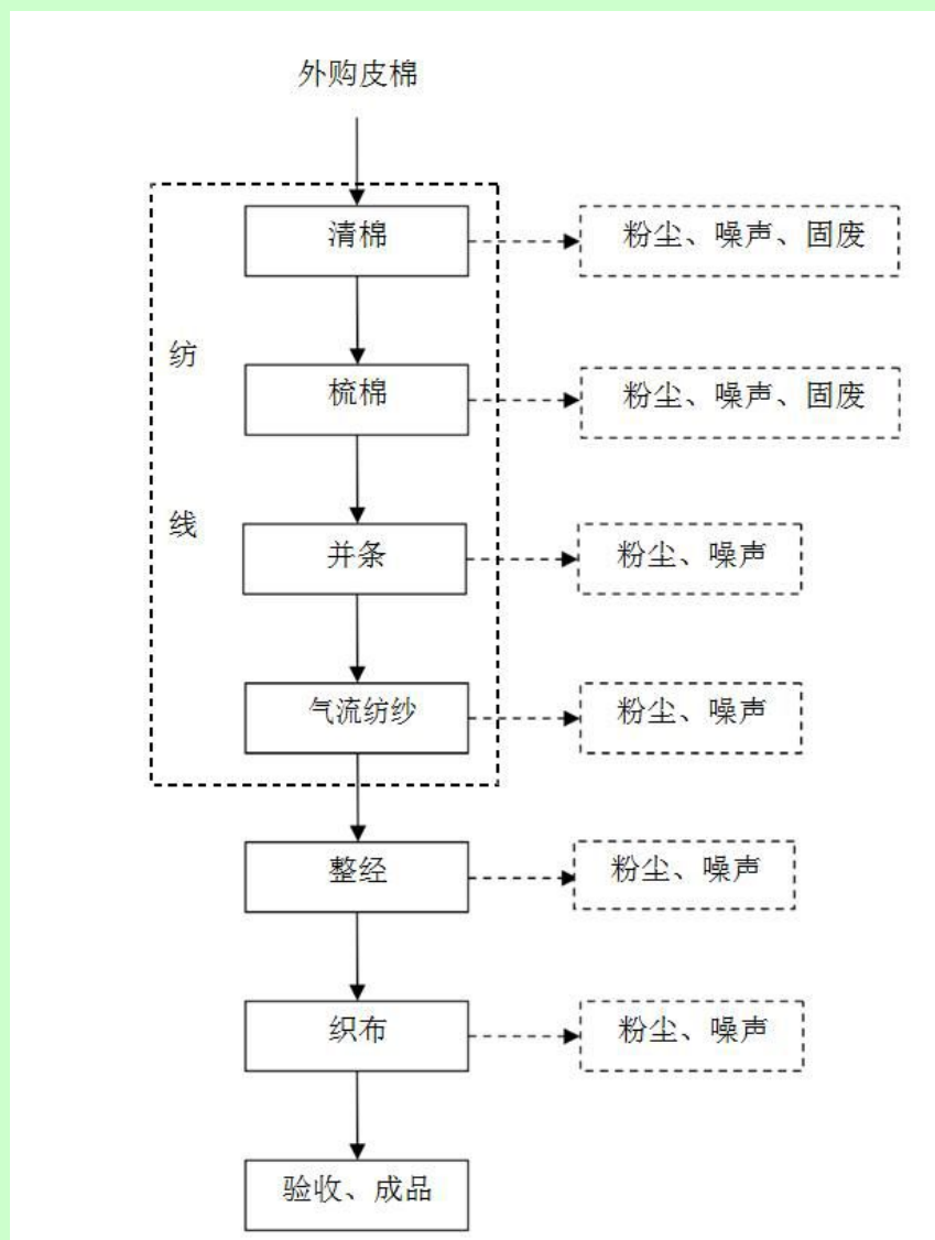
图 2 项目工艺流程及产污环节图
