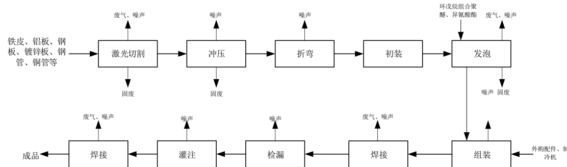
图2-1 本项目工艺流程及产排污节点图
