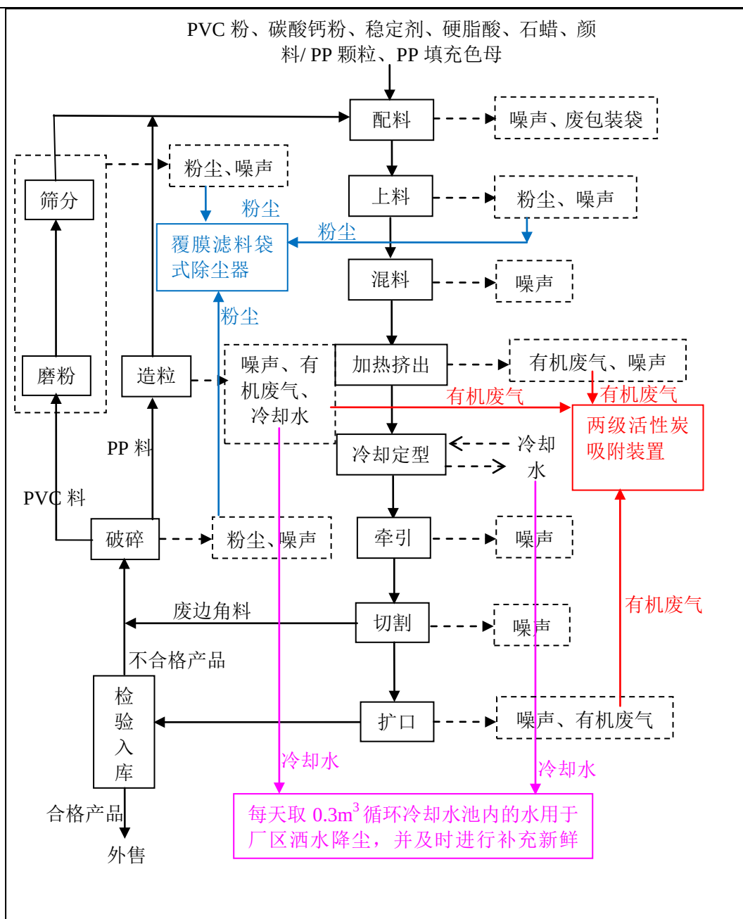
图 4 运营期工艺流程及产污环节示意图
