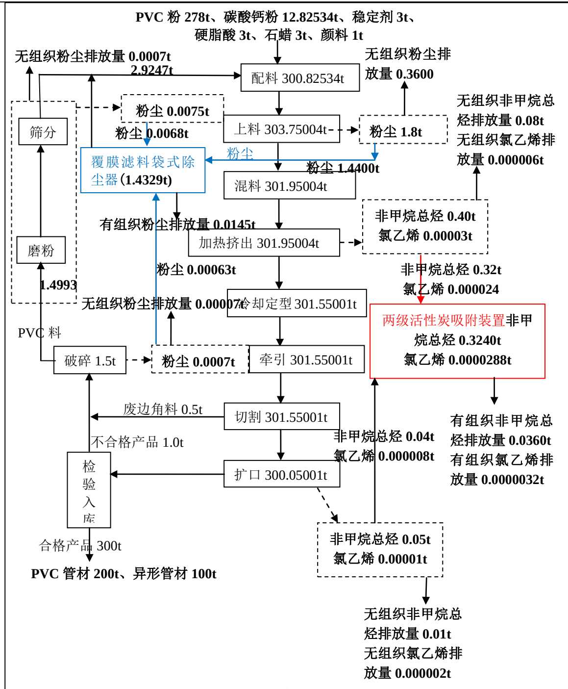
图 2 PVC 管材、异形管材物料平衡
