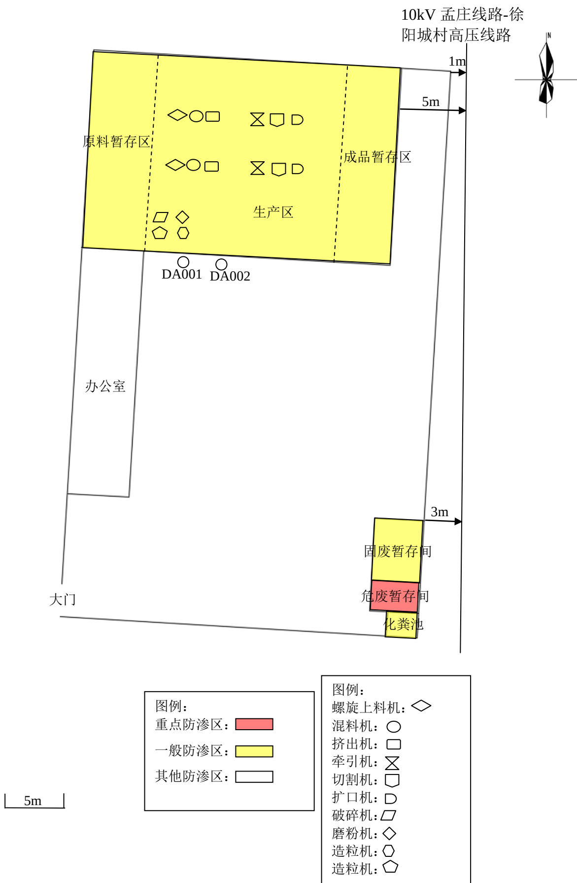
附图 4 项目厂区分区防渗图
