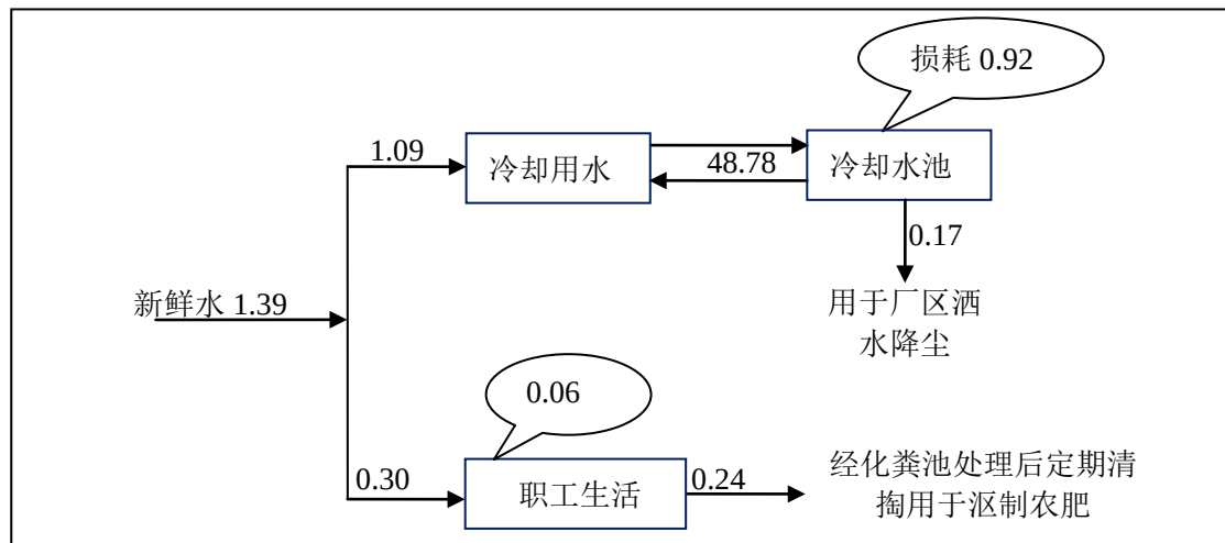
图 3 本项目水平衡图 单位: \text{m}^3/\text{d}
