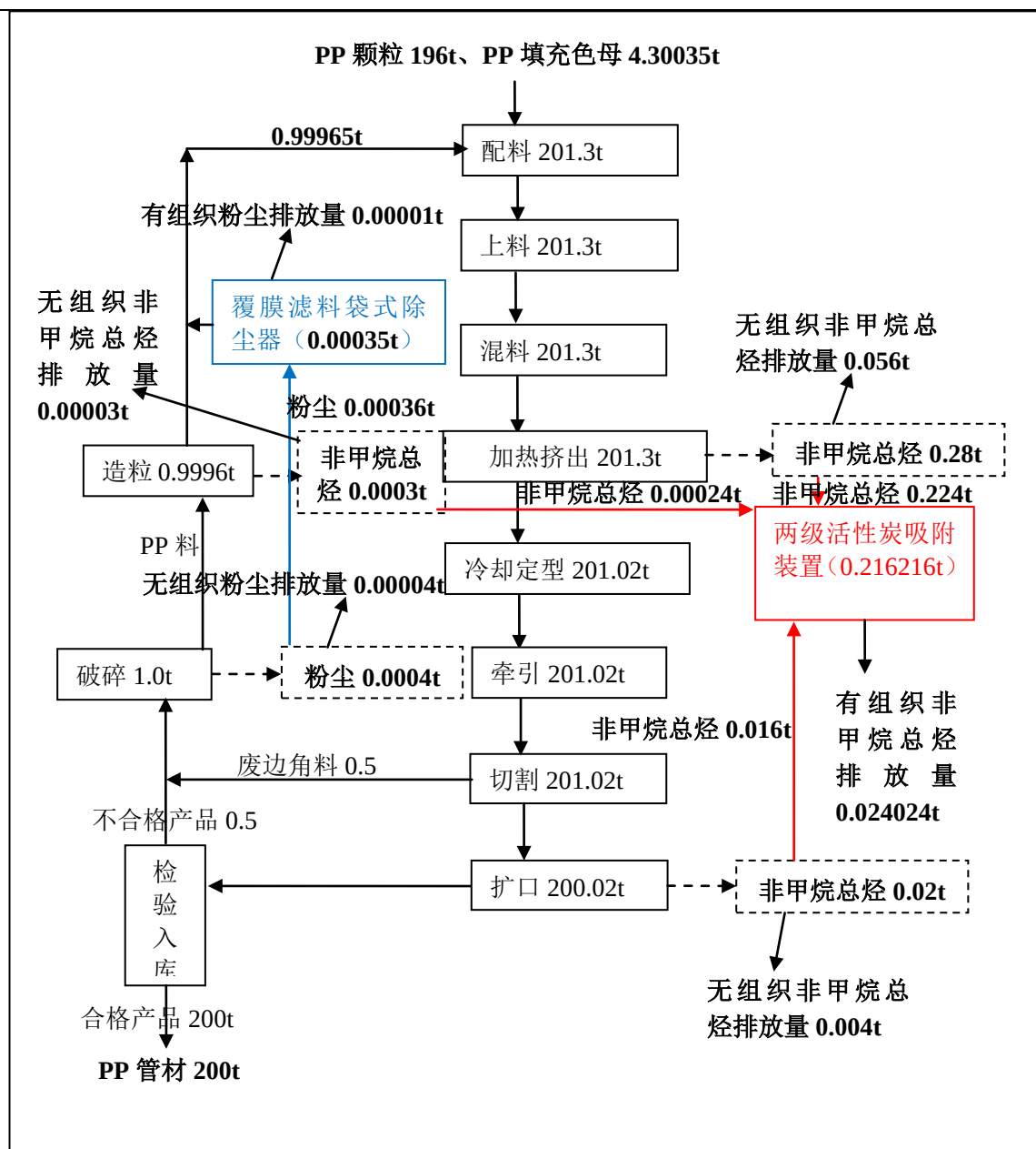
图 1 PP 管材物料平衡
